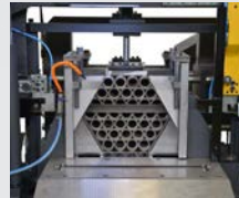
Demet Kesim Çeneleri
