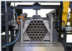
Paket Kesim Mengeneri
